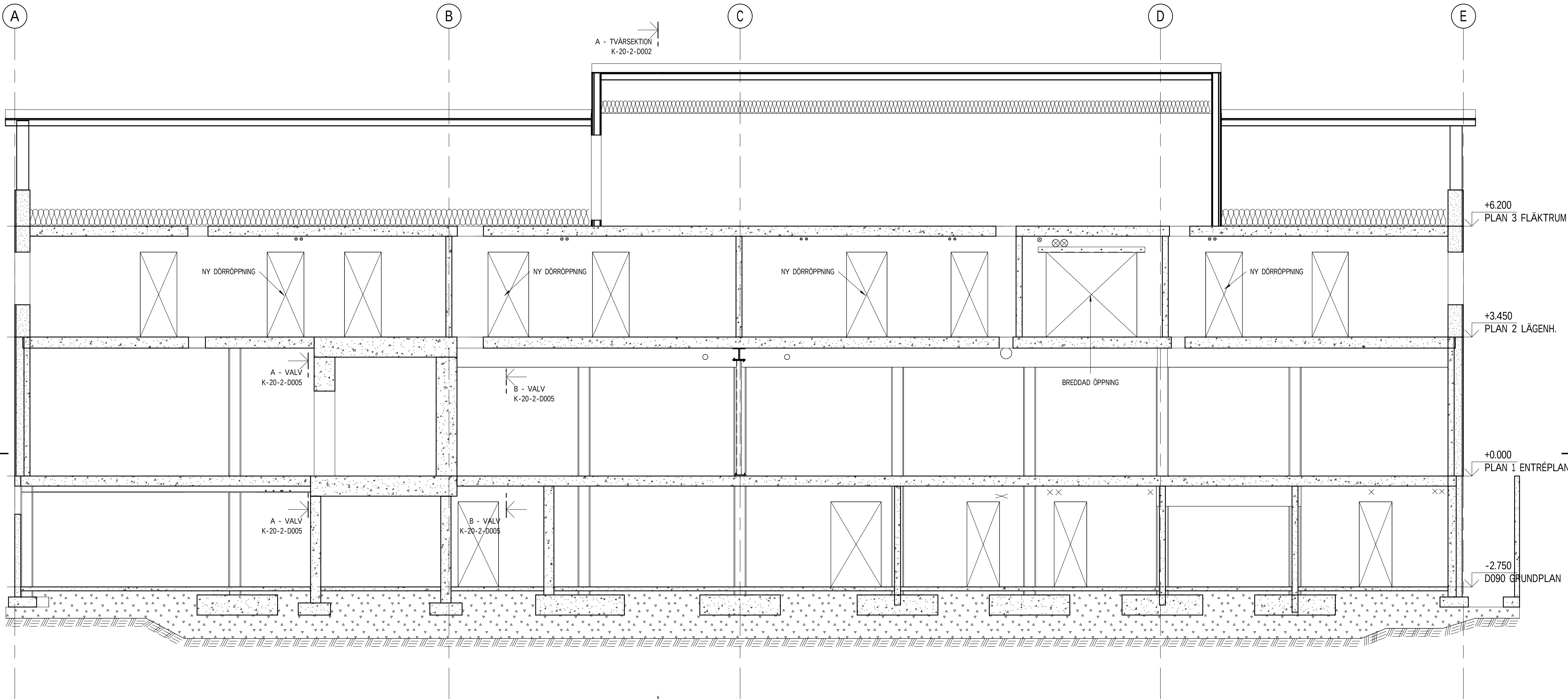
A - LÄNGDSEKTION 1 : 50
